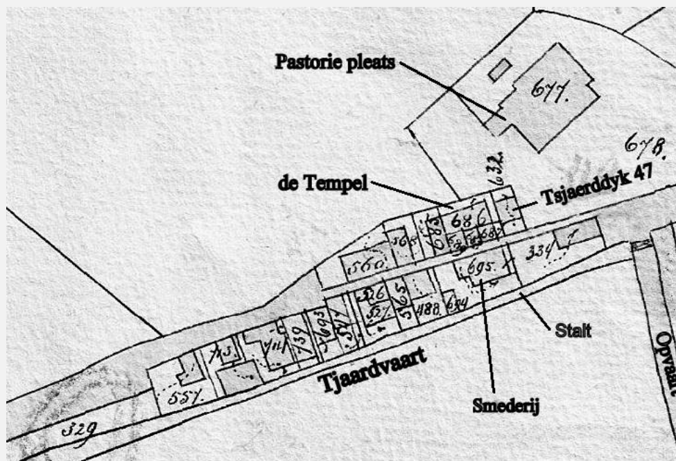
Folsgeare 1887
